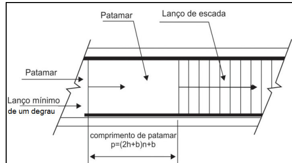
Figura 6 - Lanço mínimo e comprimento de patamar
