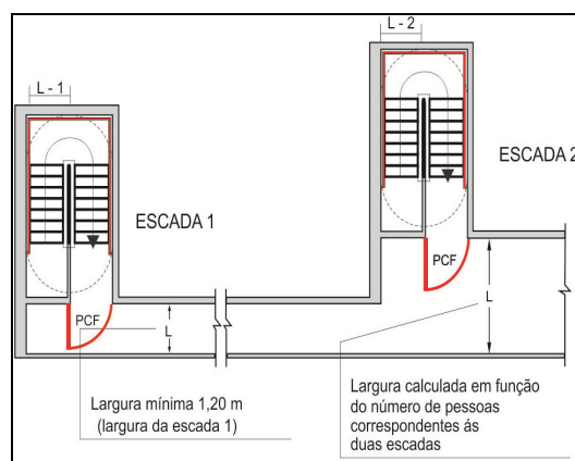
Figura 19 - Dimensionamento de corredores de descarga
