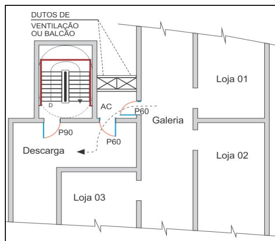
Figura 20 - Acesso de galeria comercial à descarga
