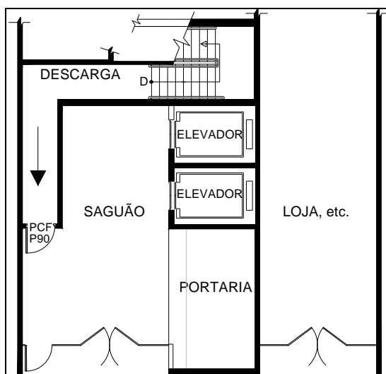
Figura 18 - Descarga através de hall térreo não enclausurado
