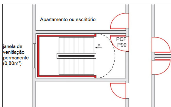
Figura 7 - Escada enclausurada protegida
